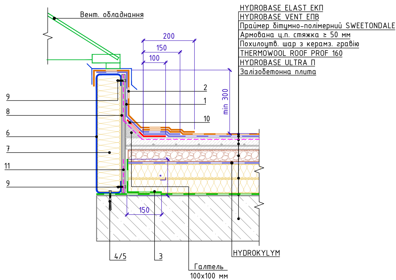
Специфікація на вузол В.3.7-2025.05
