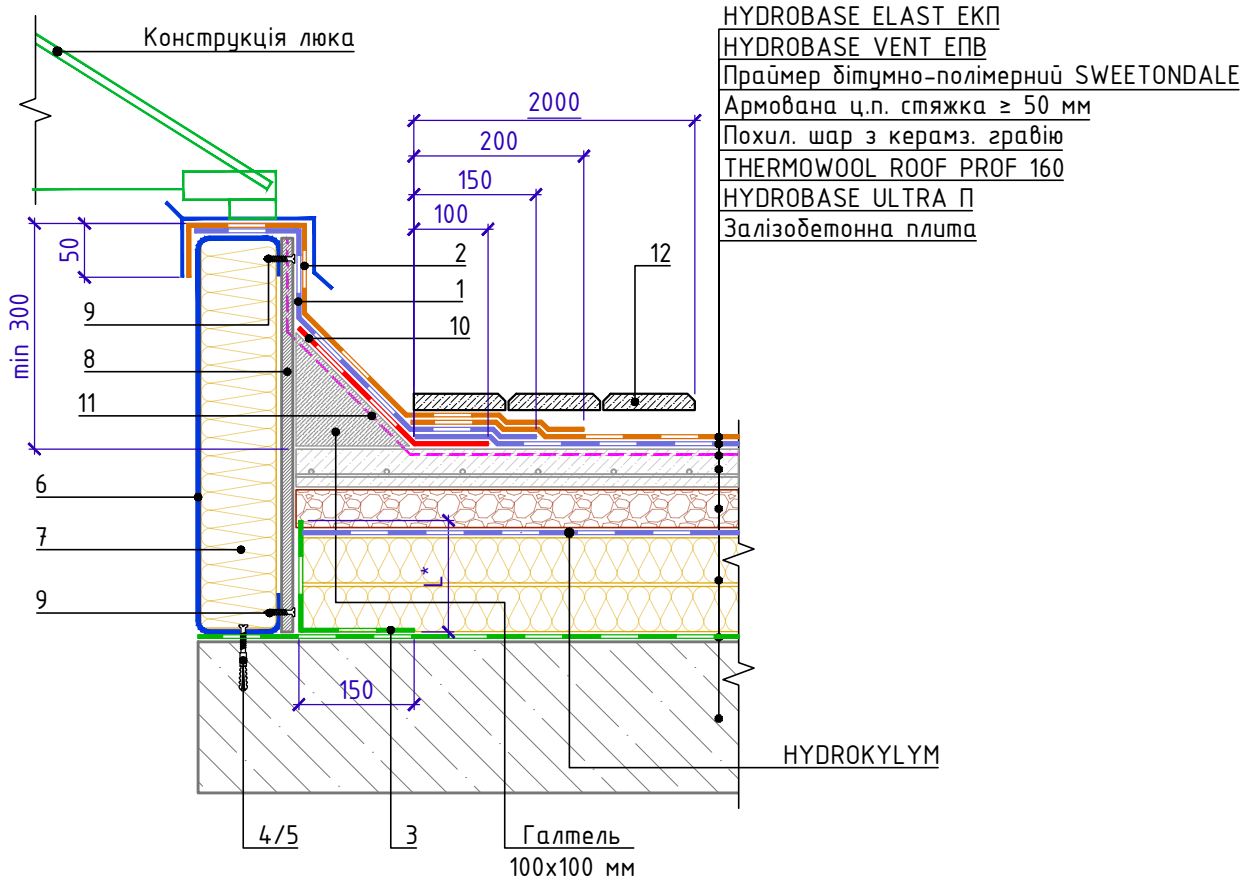
Специфікація на вузол В.7.3-2025.05
