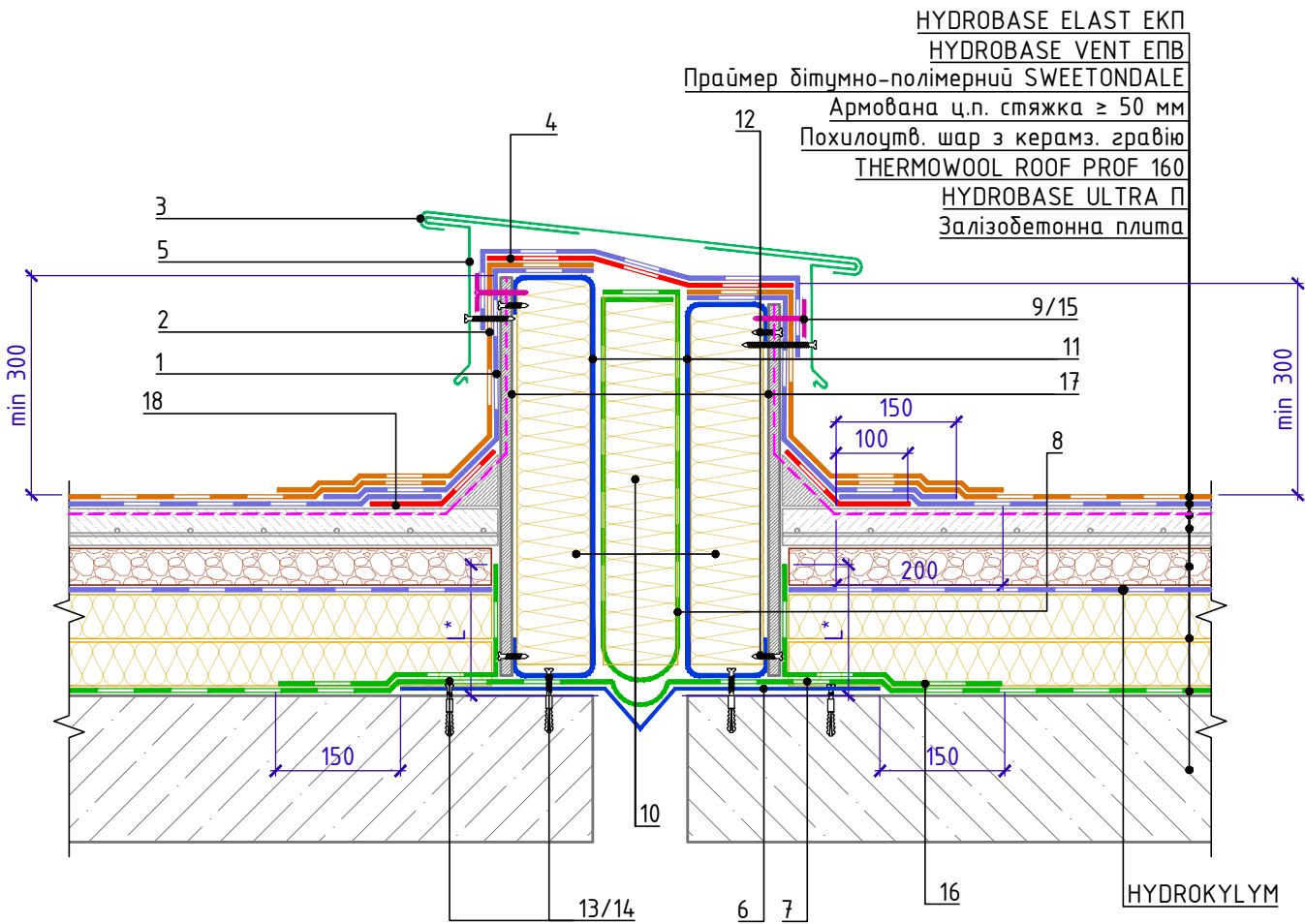
Деформаційний шов. Варіант 3
