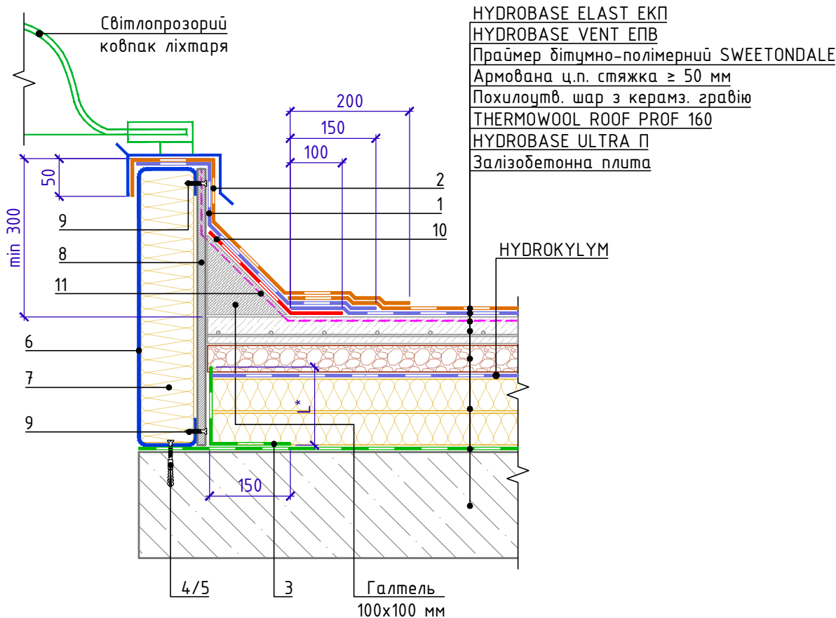
Специфікація на вузол В.9.1-2025.05
