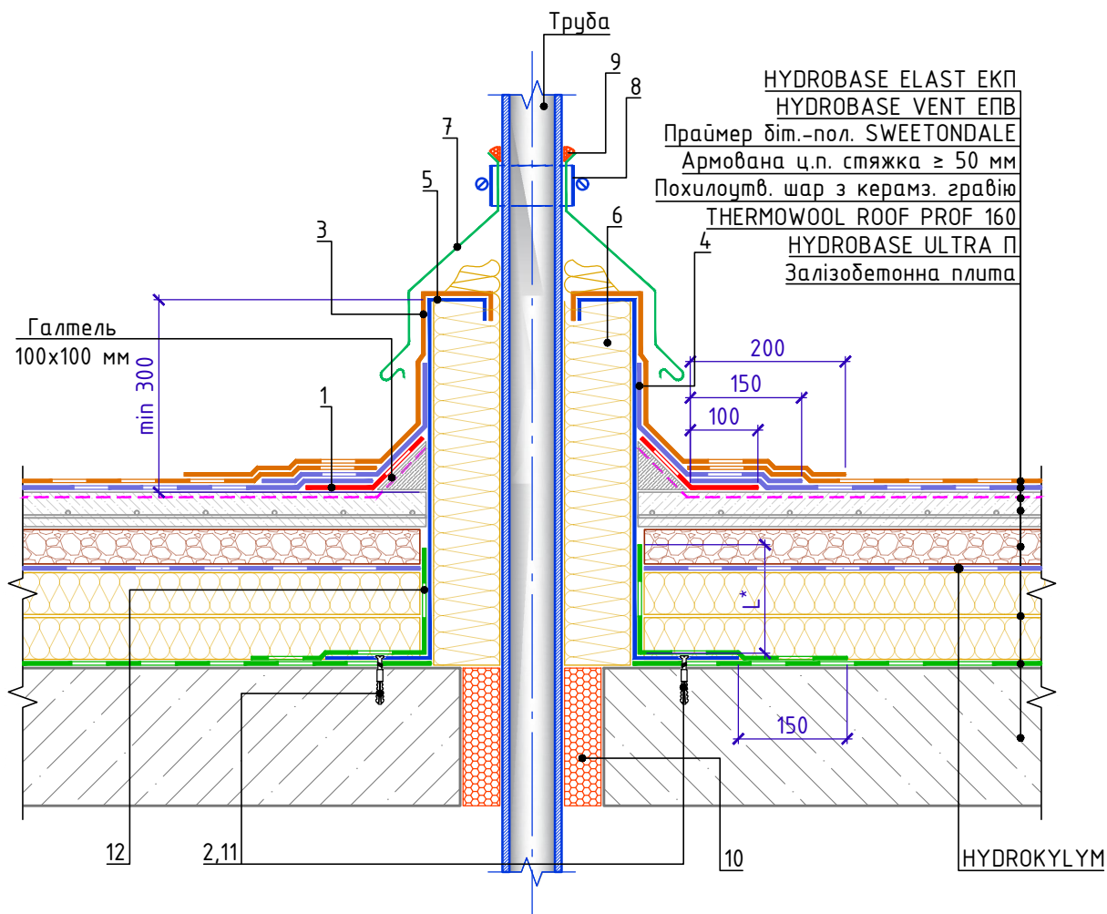
Специфікація на вузол B.3.3-2025.05
