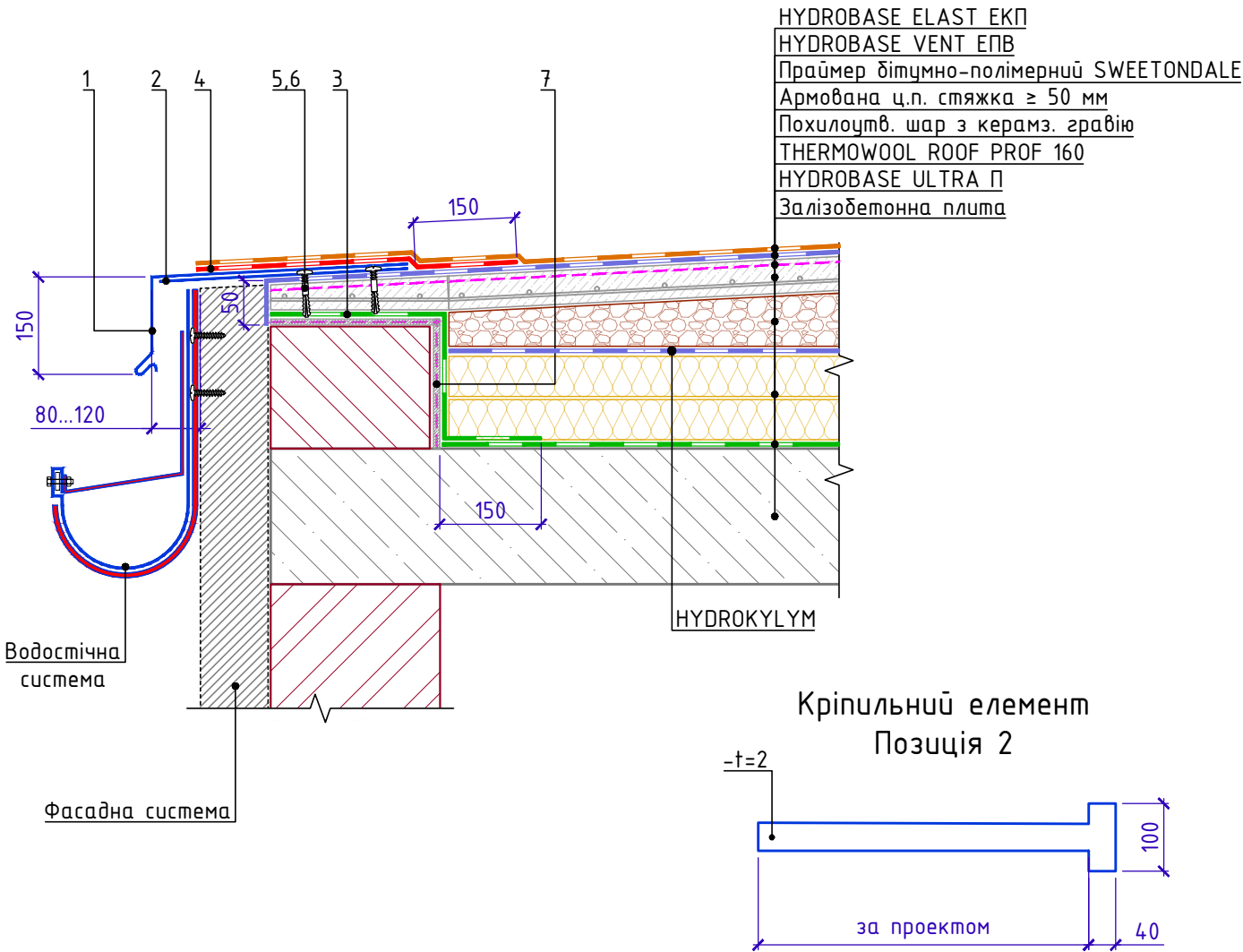
Специфікація на вузол В.1.3-2025.05
