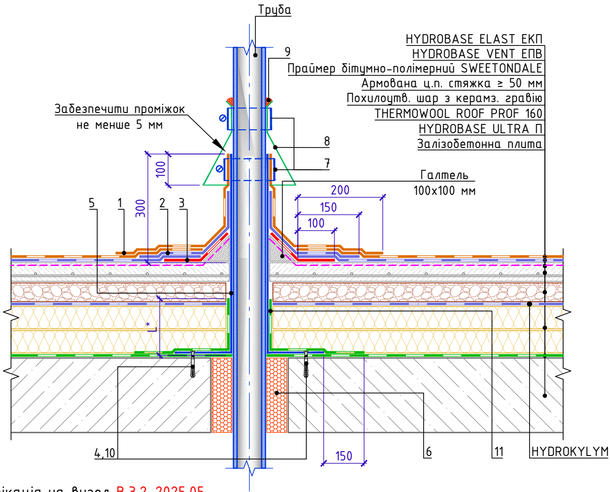
Специфікація на вузол В.3.2-2025.05
